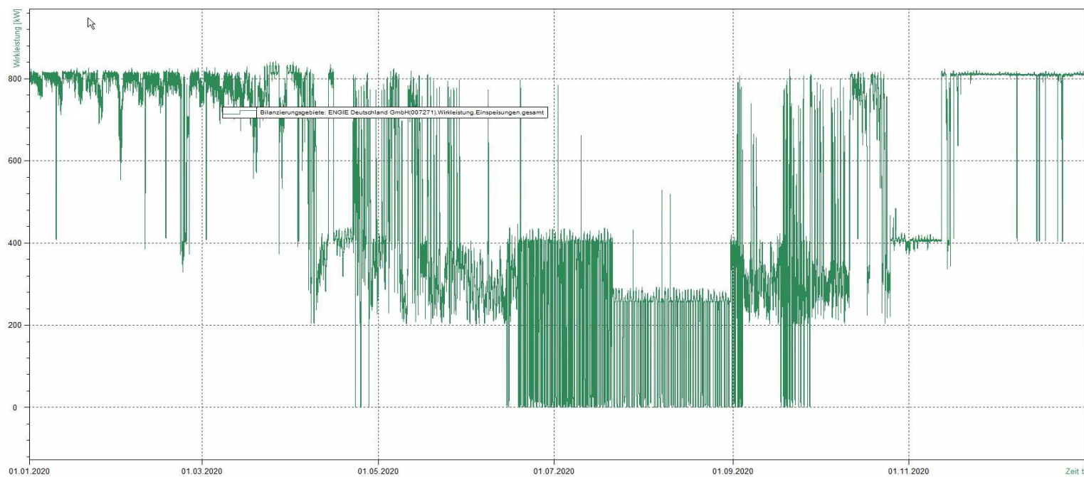
Bild 3: Summe aller Einspeisungen NS
